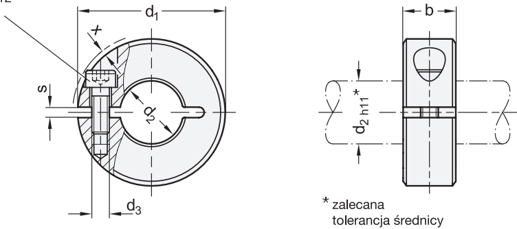
Śruba z łbem gniazdowym DIN 912
